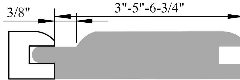
FL # 519 3/4"x 4"- 8"
