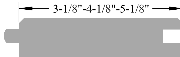
FL # 508 3/4"x 4"- 6"
