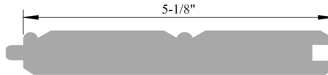
FL # 353 1"x 6"
